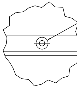
Ø.172 THRU TYP Ø.375 FIRST & SECOND WALLS TYP
